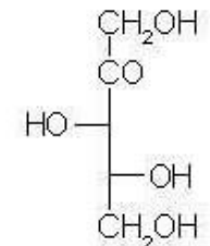
D-xylulosa
