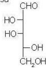
D-lyxosa
