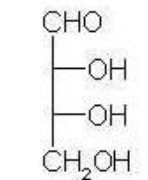
D-erythrosa
