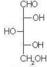
D-xylosa
