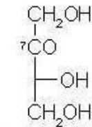
D-erythrulosa
