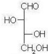
D-threosa
