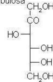
D-fruktosa
