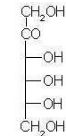
D-psikosa
