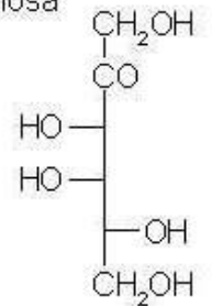
D-tagatosa
