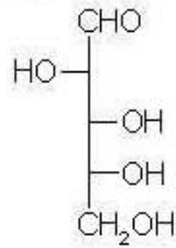
D-arabinosa
