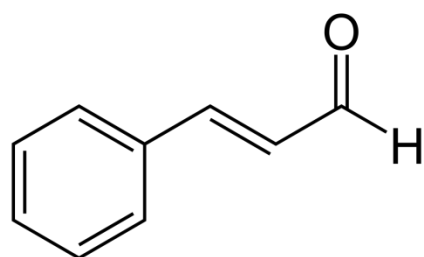
cinnamaldehyd
