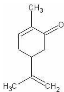
karvon
