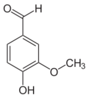
vanilin
