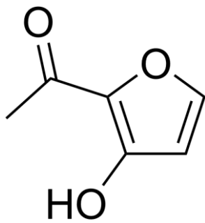
isomaltol
