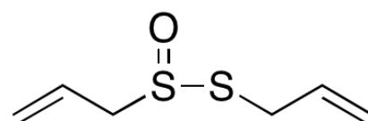
allicin
