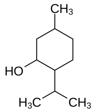
menthol
