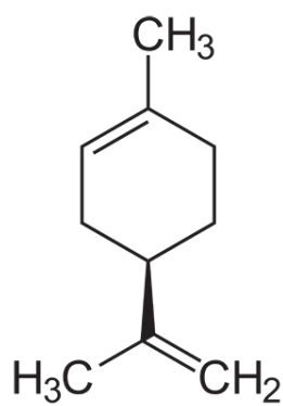
limonen
