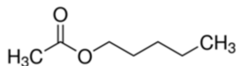
pentylacetát
