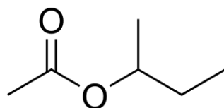
isobutylacetát
