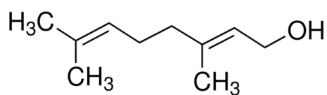
geraniol
