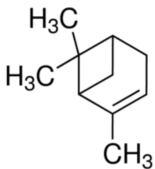
\alpha - pinen
