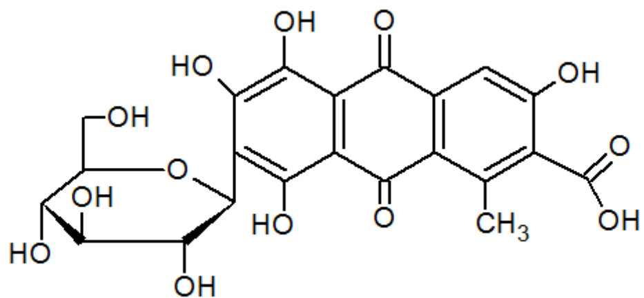
struktura karminové kyseliny
