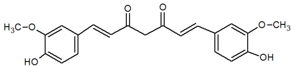
struktura kurkuminu
