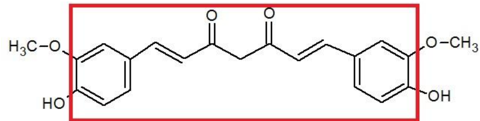
zvýrazněný chromofor kurkuminu
