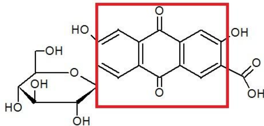
zvýrazněný chromofor kurkuminu
