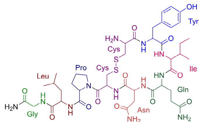
Obrázek 4: oxytocin Cys-Tyr-Ile-Gln-Asn-Cys-Pro-Leu-Gly-NH 2
